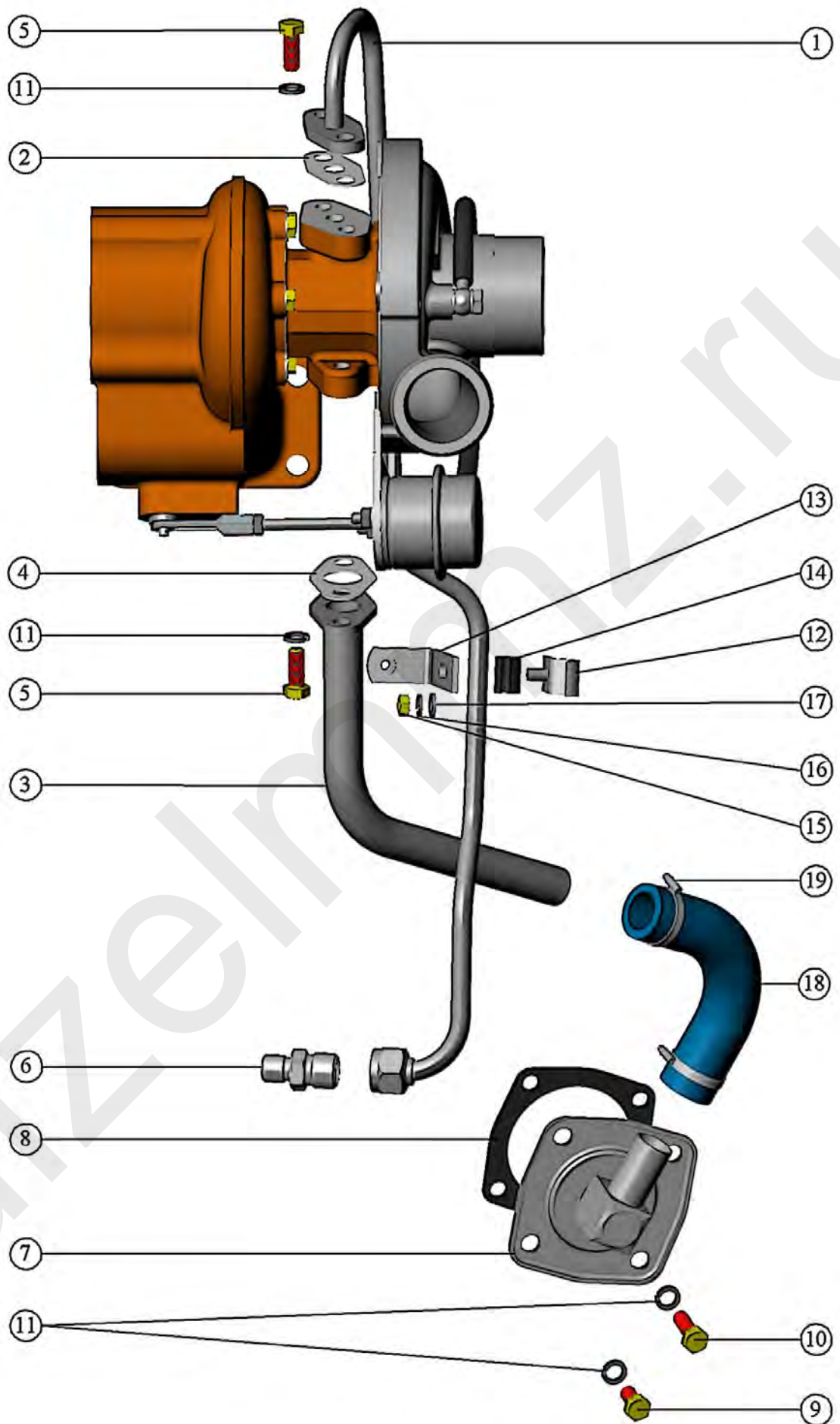
Рис. 13 Маслопроводы турбокомпрессора.
