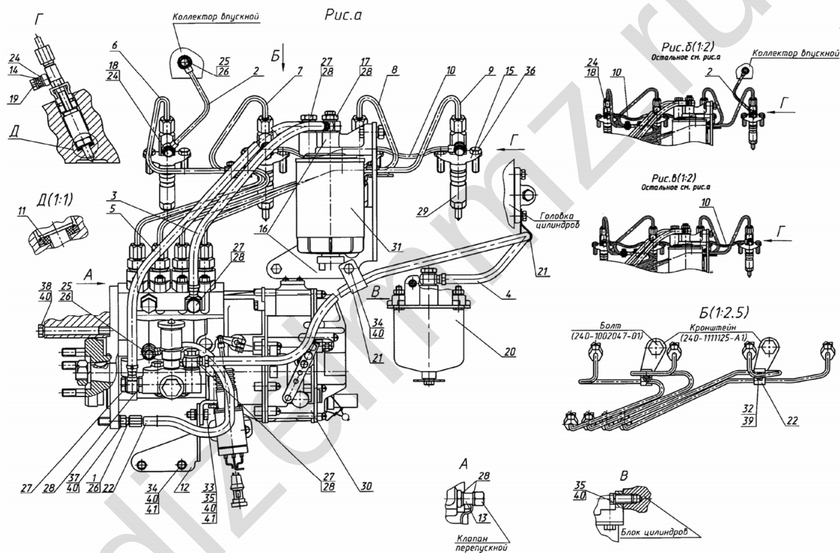
Рис. 9 Топливные трубопроводы и установка топливной аппаратуры
