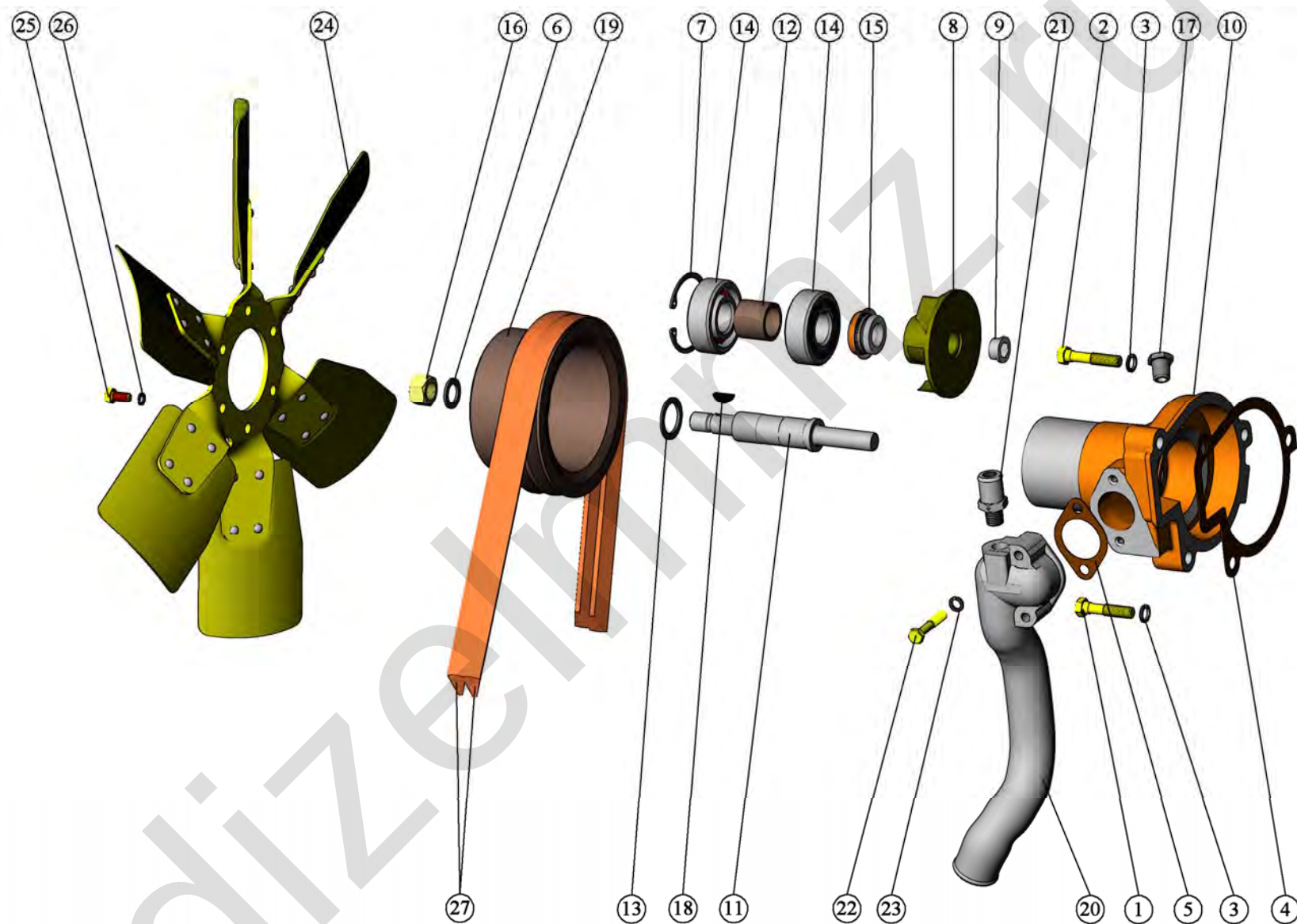
Рис. 14 Установка водяного насоса. Установка вентилятора
