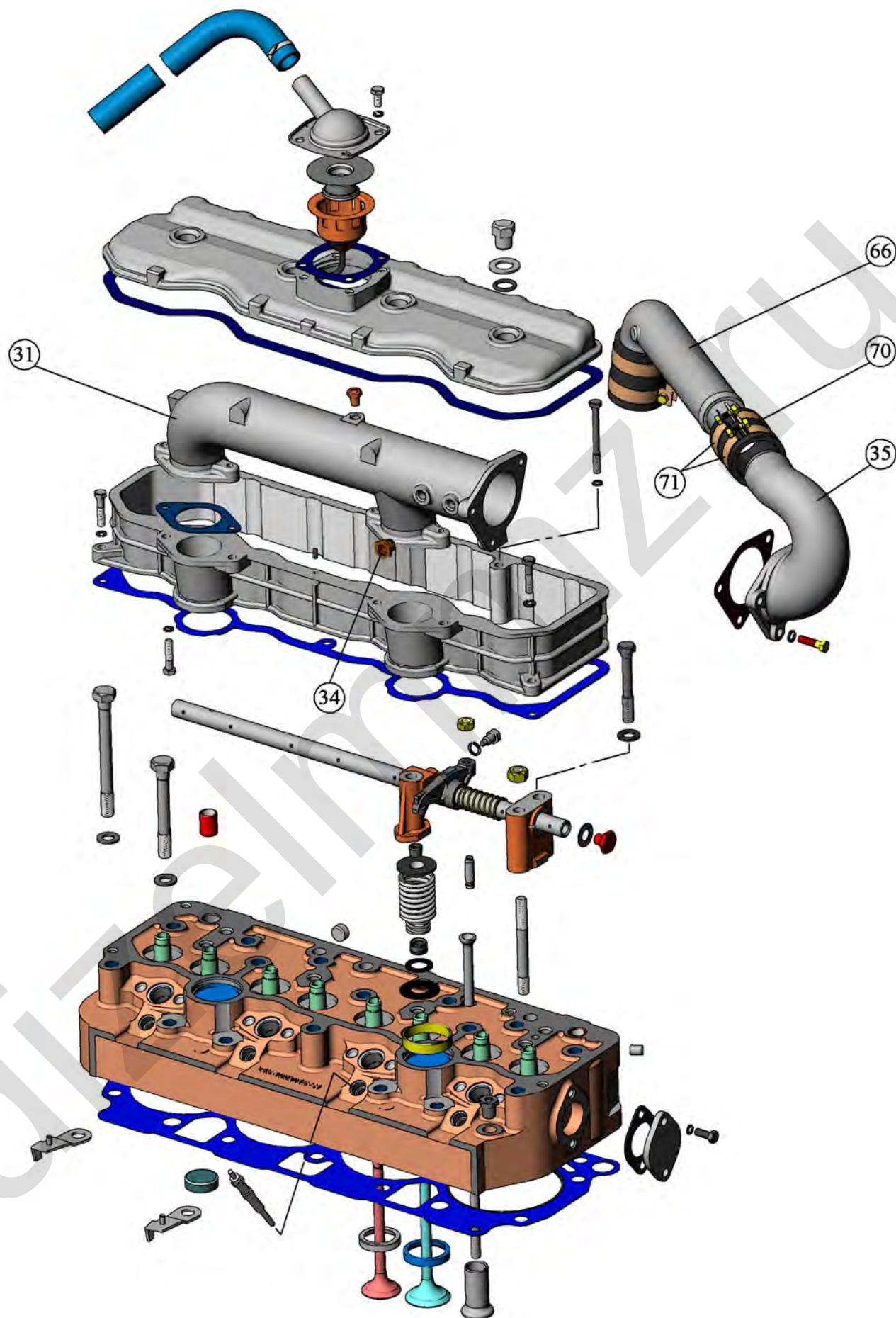
Рис. 2а Установка головки цилиндров и впускного тракта. Клапаны и толкатели клапанов (для дизеля Д-246.2) (остальное смотрите рис. 2)
