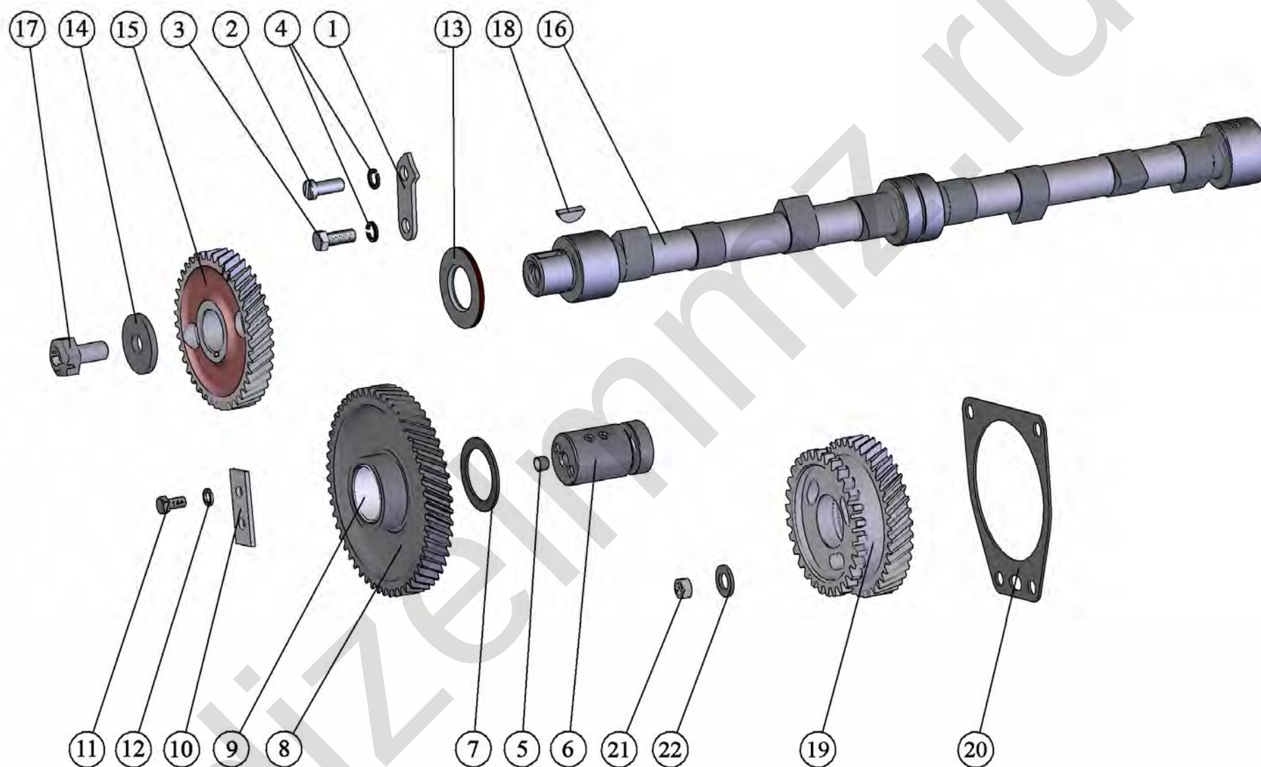
Рис. 4 Распределительный механизм
