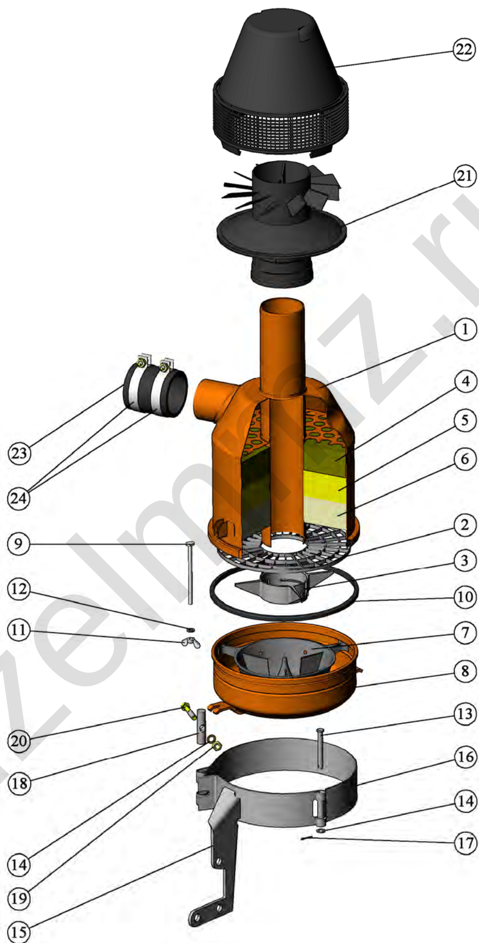
Рис. 10 Установка воздухоочистителя
