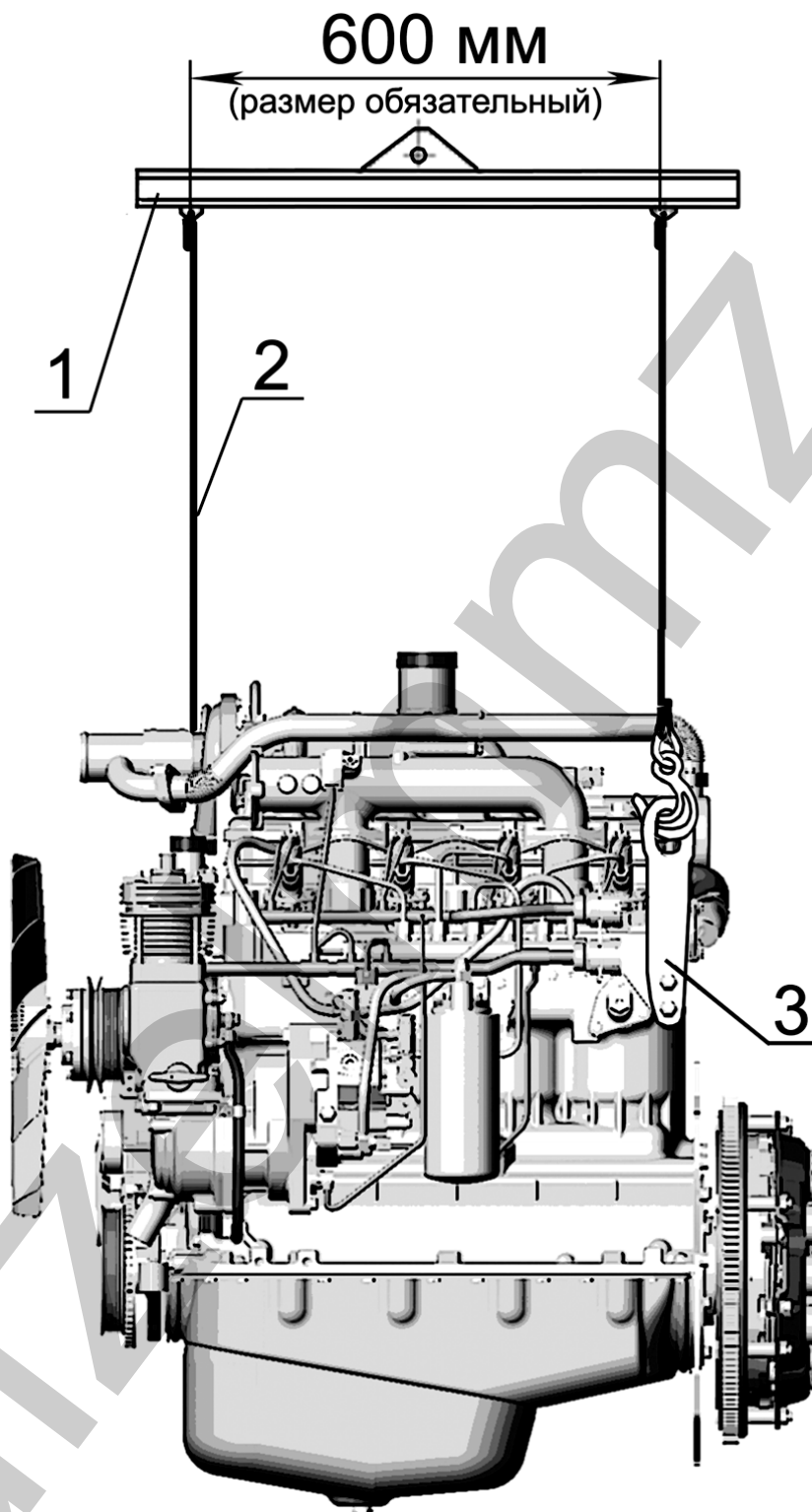
Рисунок И.1 – Схема строповки дизеля.
