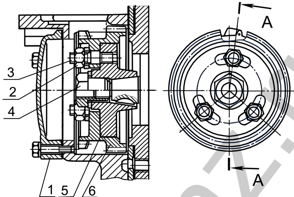
Рисунок Д.6 - Привод редуктора.
