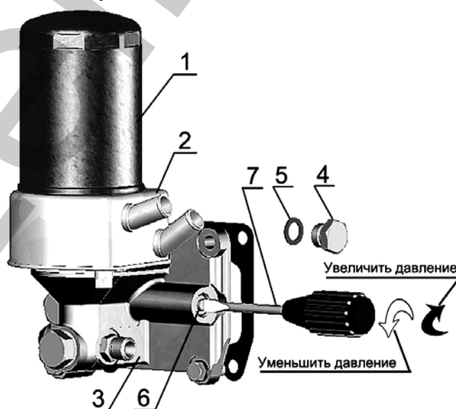
Рисунок 19 – Регулировка давления масла.
