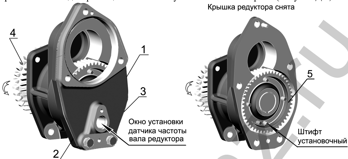
Рисунок Д.4– Редуктор привода ТНВД.
