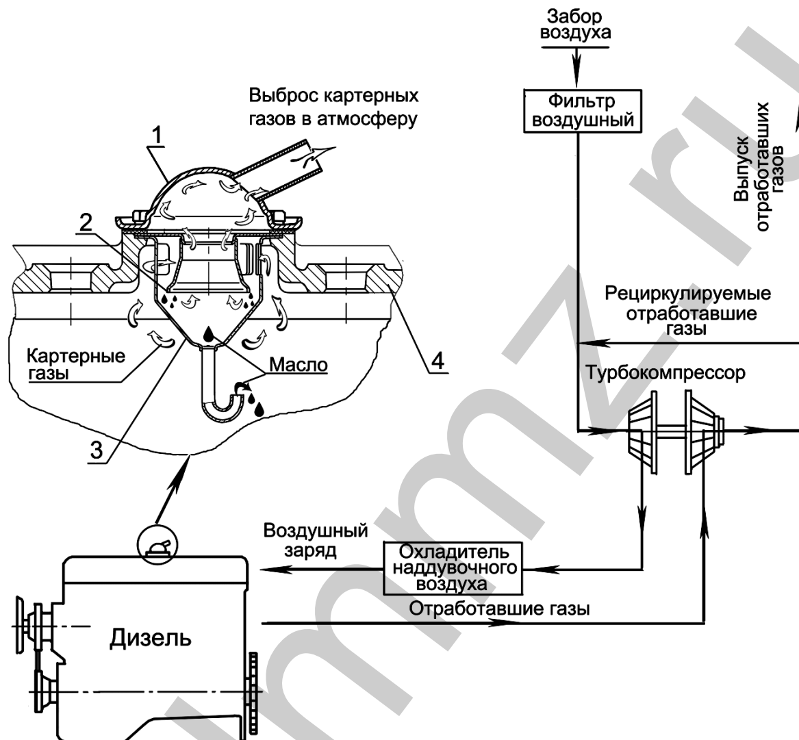
Рисунок – 14 Схема газообмена дизеля.
