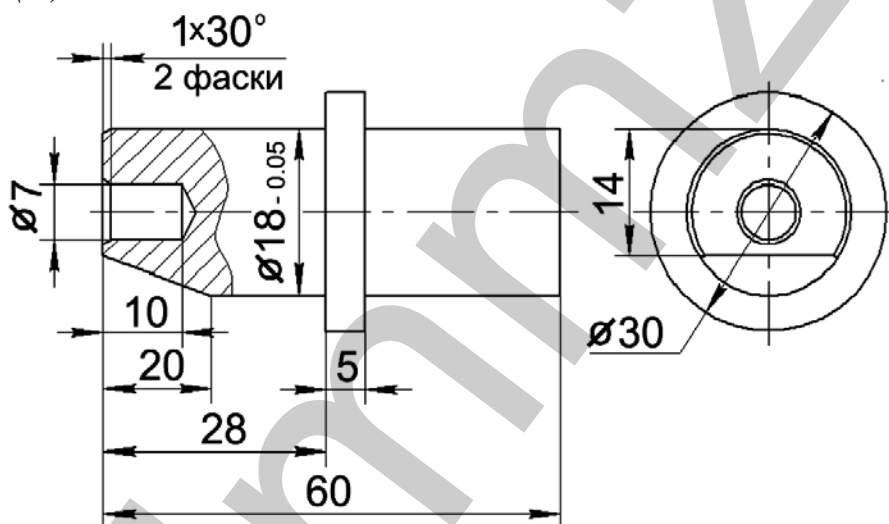
Рисунок Д.1 – Приспособление для фиксации установочного штифта.
