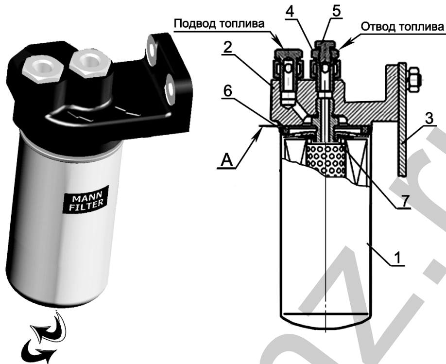
Рисунок 22- Замена фильтра тонкой очистки топлива.
