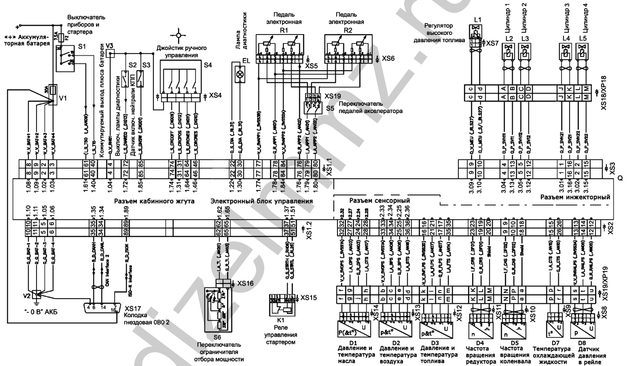
Структурная электрическая схема электронного управления дизелем
