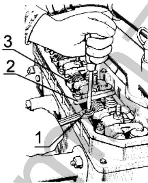
1 – винт регулировочный; 2 – щуп; 3 – контргайка. Рисунок 26 - Регулировка зазора в клапанах.
