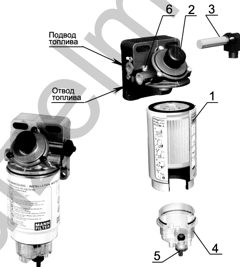
1 – фильтр грубой очистки топлива; 2 – ручной топливоподкачивающий насос; 3 – подогреватель топлива; 4 – влагоборник; 5 – кран выпуска воды; 6 – пробка для выпуска воздуха.
